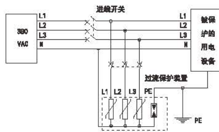
三相四线 (TT) 系统 PHL-TA-40/440/3P+1
