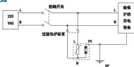
单相 (TT) 系统 PHL-TA-40/440/1P+1
